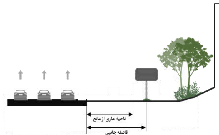
ب- تأمین فاصله عاری از مانع و عدم نیاز به نصب حفاظ طولی
