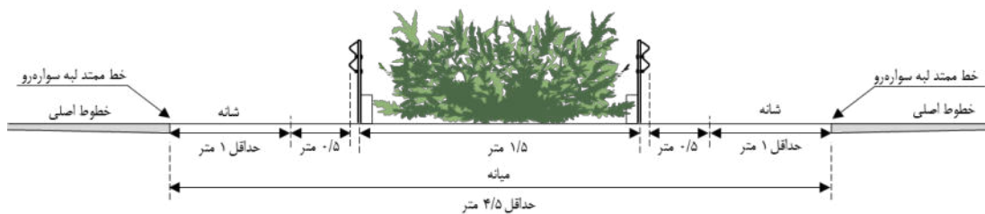
شکل ۴-۱۱- مشخصات هندسی میانه با حفاظ طولی انعطاف‌پذیر در آزادراه
