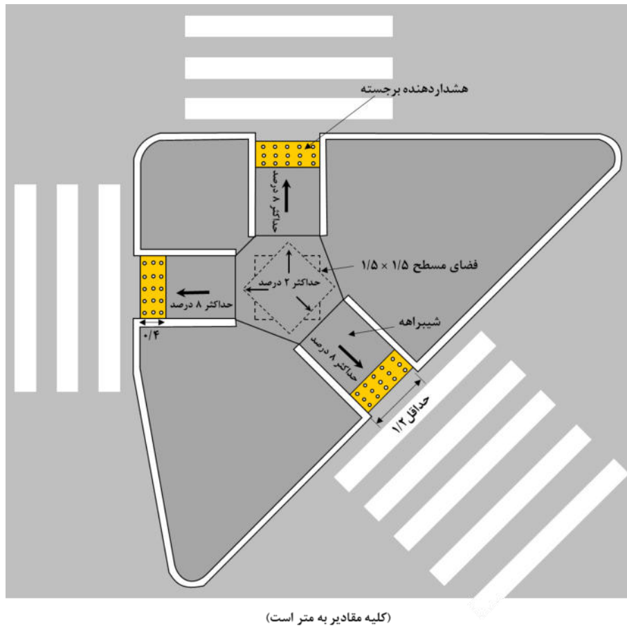
شکل ۳-۱۹- مشخصات هندسی مسیر حرکت عابران پیاده در جزیره‌های مثلثی شکل دارای شیرابه
