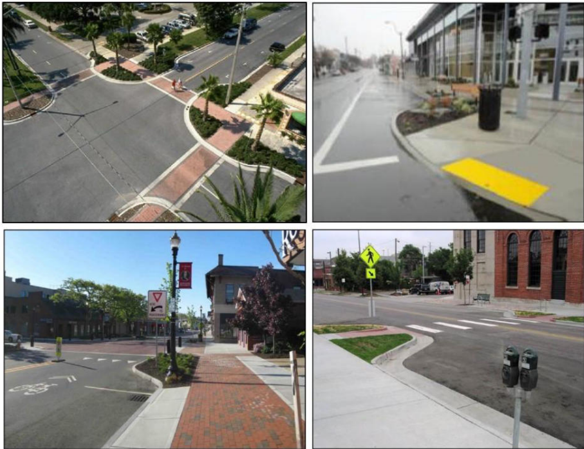
شکل ۳-۷- نمونه‌های اجرا شده از پیش‌آمدگی جدول
