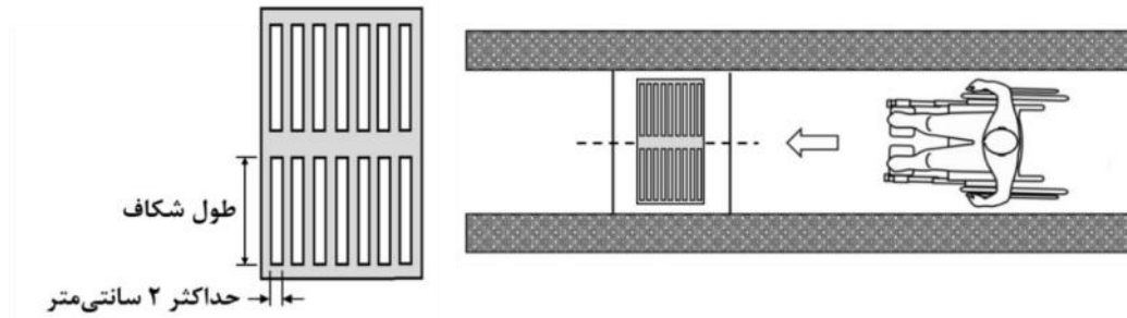
شکل ۸-۲- نحوه نصب دریچه‌های جمع‌آوری آب‌های سطحی در سطح پیاده‌رو
